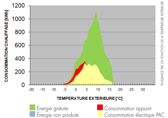
RÉPARTITION DES PRODUCTIONS DE CHAUFFAGE (données station de référence)
