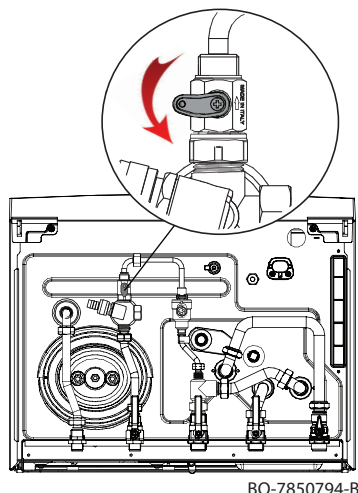
Fig.21 Remplissage de l'installation
