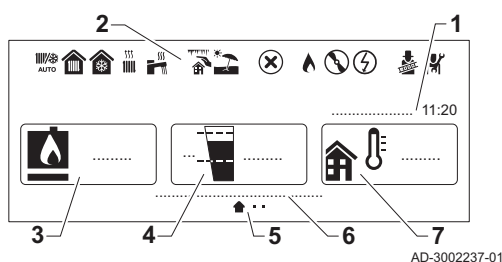
Fig.2 Description de l'écran d'accueil
