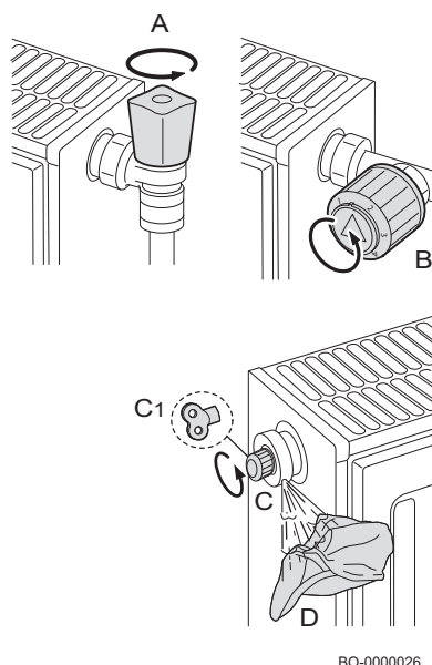
Fig.22 Purge de l'installation
